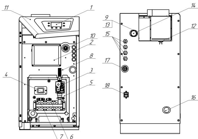
Рис. 1. Конструкция котла
